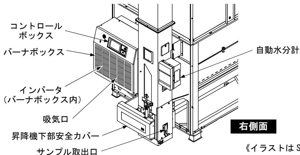
図 3 機械全体図 (1)
